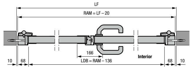
Ușă alăturată cu 2 canaturi și toc bloc din aluminiu, profil de tip 2 Montaj în deschidere
