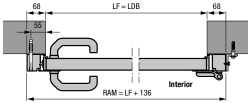
Ușă alăturată cu toc bloc din aluminiu, profil de tip 1 Montare în spatele golului din zidărie
