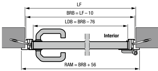
Ușă alăturată cu toc de colț din aluminiu, tip profil 1 sau 2 Deschidere la exterior
