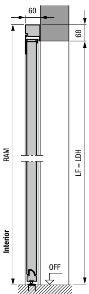
Ușă alăturată cu toc bloc din aluminiu, profil de tip 2 Montare în spatele golului din zidărie
