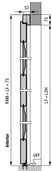
Ușă alăturată din lemn masiv Montare în spatele golului din zidărie
