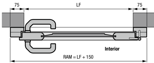
Ușă alăturată din lemn masiv Montare în spatele golului din zidărie
