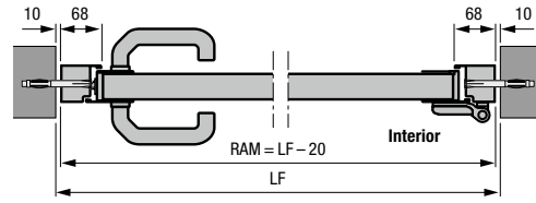
Ușă alăturată cu toc bloc din aluminiu, profil de tip 2 Montaj în deschidere
